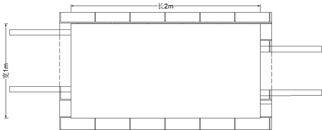
沉沙池平面示意图
