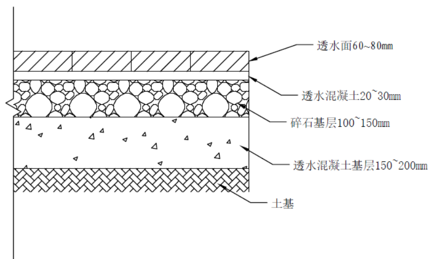
透水砖铺装示意图
