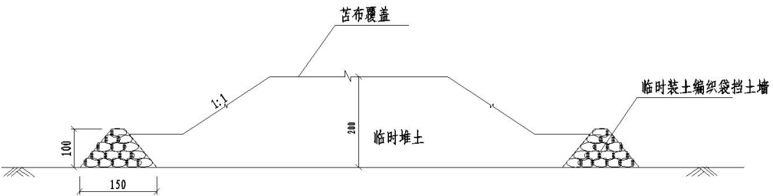
临时堆土防护措施剖面示意图 装土编织袋挡墙单位工程量表
