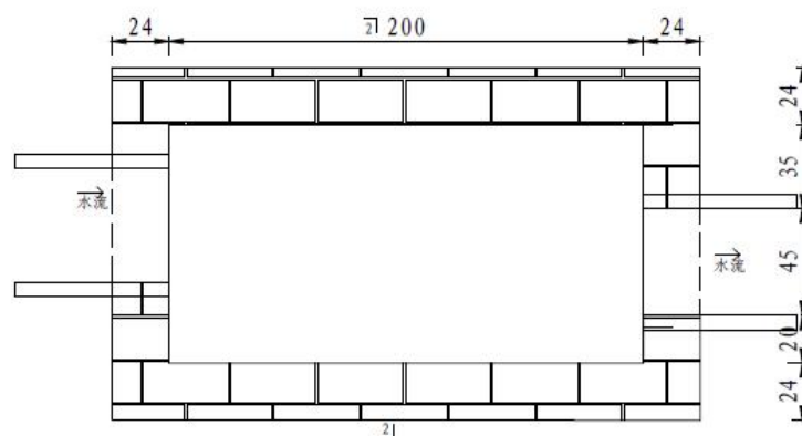
主体工程防治区布设沉沙池 4 座，工程量为：土方开挖 50.84m 3 ，土方回填 27.36m 3 ，M7.5 砌砖 10m 3 ，M10 水泥沙浆抹面 42.68m 2 ，C20 砼 1.48m 3 。
